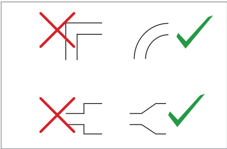
Figure 18: éviter les coudes à 90° et les adaptateurs trop réducteurs
